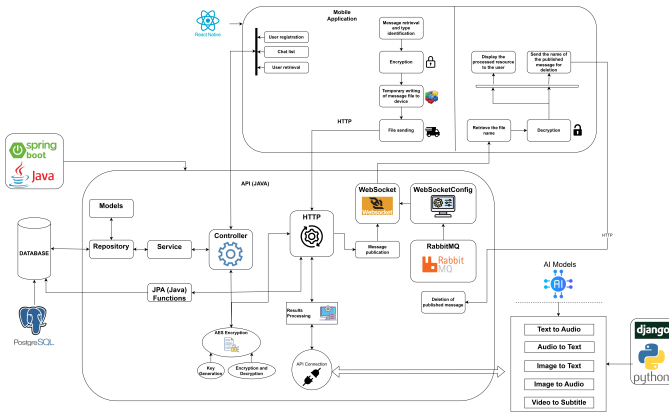
Figura 1. Arquitectura del sistema de mensajería móvil inclusiva. Se muestran la capa de presentación (React Native), la capa de negocio (API REST Spring Boot y API IA Django con RabbitMQ), la capa de persistencia (PostgreSQL) y los módulos de conversión multimodal (TTS, STT, imagen a texto, imagen a audio, video a subtítulo) con cifrado AES de extremo a extremo.
