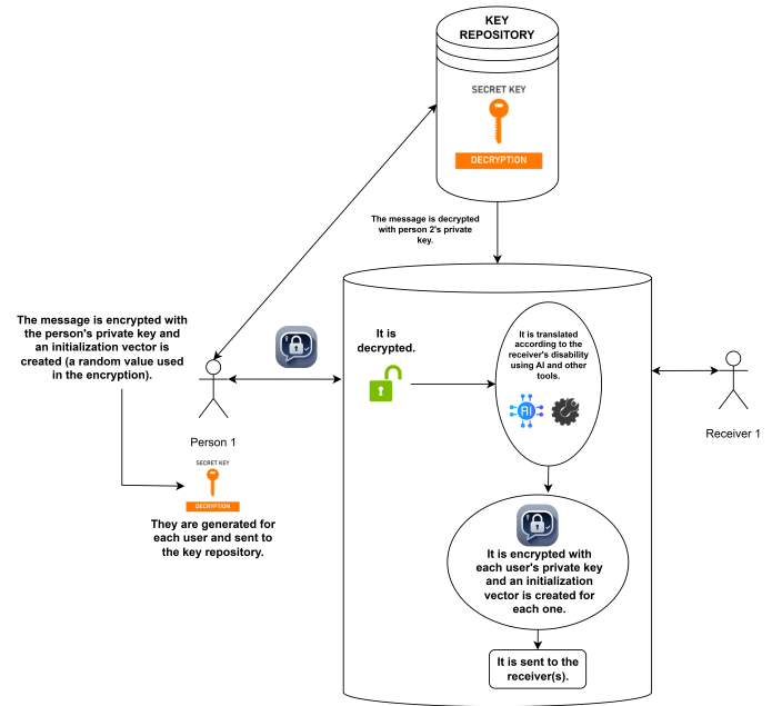
Figura 2. Flujo de comunicación segura y accesible: cifrado con claves privadas y adaptación del mensaje mediante inteligencia artificial según el perfil sensorial del receptor. El mensaje se cifra en origen, se descifra en el servidor para su conversión accesible y se re-cifra antes de la entrega final.
